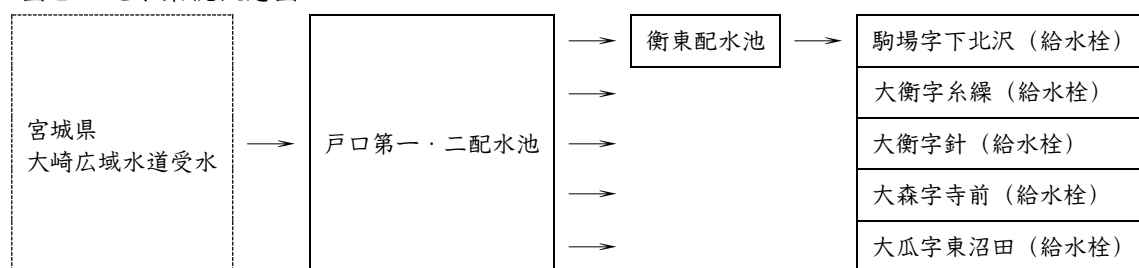
図1：配水系統概念図
